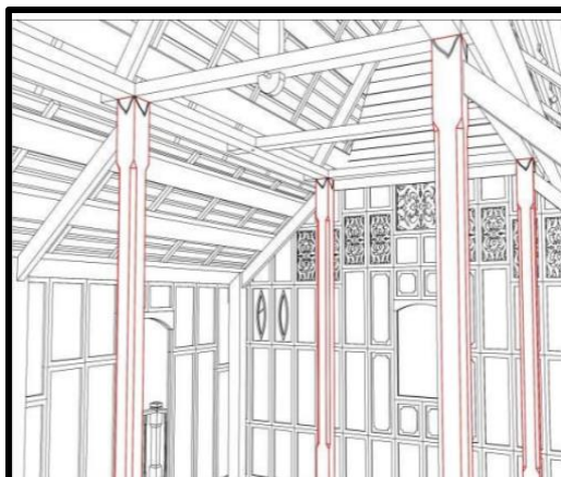
Rajah 9 Lakaran rekabentuk tiang seri Rumah Tele
